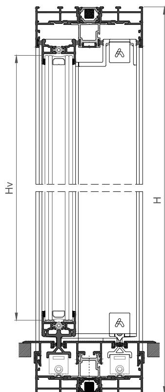
SECCIÓN B-B SECTION B-B
