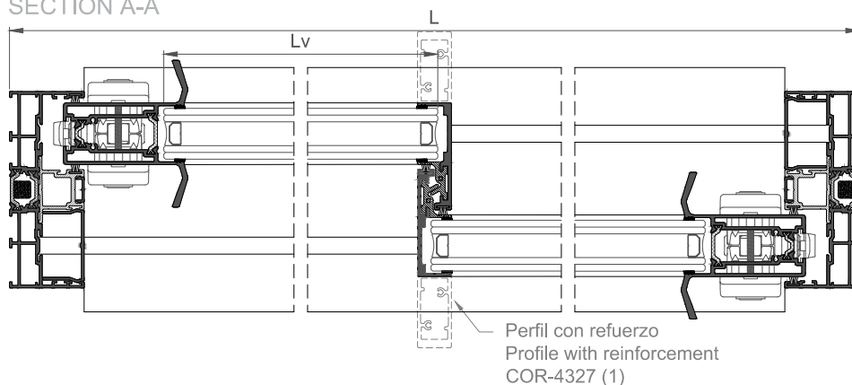
SECCIÓN A-A SECTION A-A
